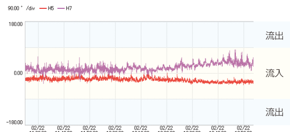
流入 / 流出判定の例 (5 次、7 次高調波が流入)
