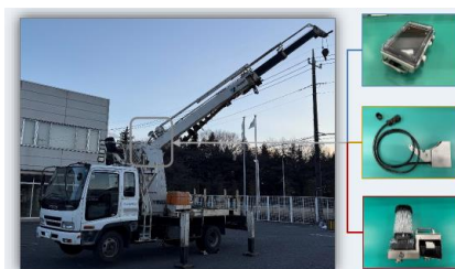
ブームウォッチャー 吊荷の荷重を入力することで、許 容範囲の確認とランプでの警告
